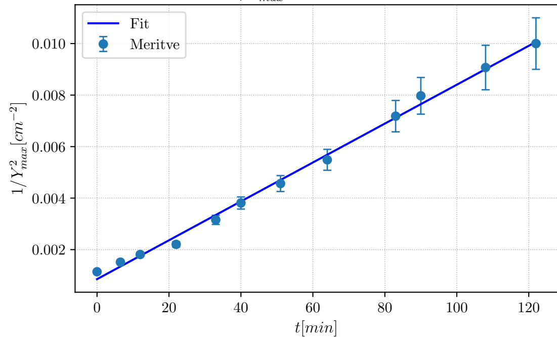
Graf 1/Y_{max}^2 v odvisnosti od časa
